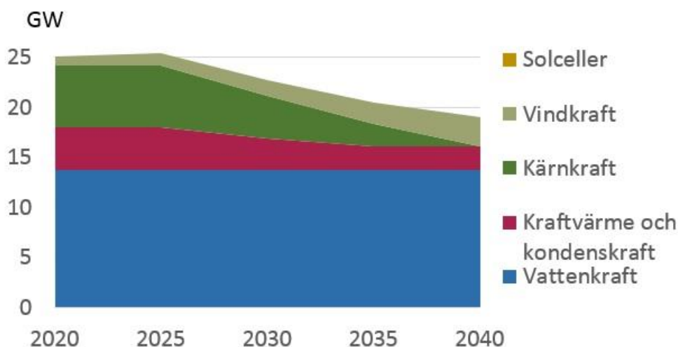
Figur 8 Produktionskapacitet i Sverige som man kan räkna med finns tillgänglig de kritiska timmarna då det nationella elnätet är ansträngt. Grafen motsvarar det scenario som Svenska Kraftnät redovisar i figur 3 i sin systemutvecklingsplan för perioden 2018 - 2027. Den tillgängliga kapaciteten som visas i grafen ska ställas i relation till den senaste vinterns maximala elanvändning, som var 25,9 GW.
